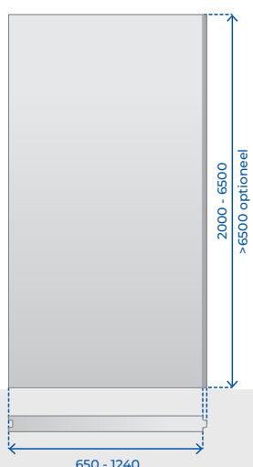
SP Standaard paneel Standard Panel
