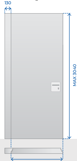
FHD Loopdeur vast aan stijl Full Height Door
