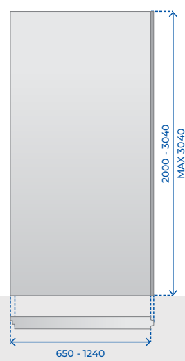
DAP Deur aanslag paneel Door Attach Panel
