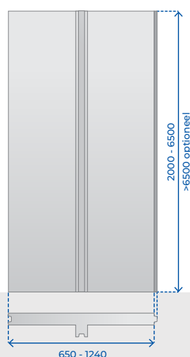
STP Enkel T-paneel Single T-Panel
