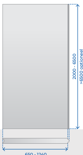
SP Standaard paneel Standard Panel
