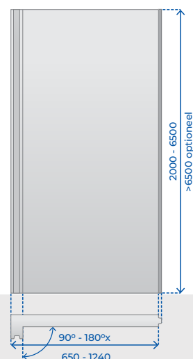
CP Hoek paneel Corner Panel
