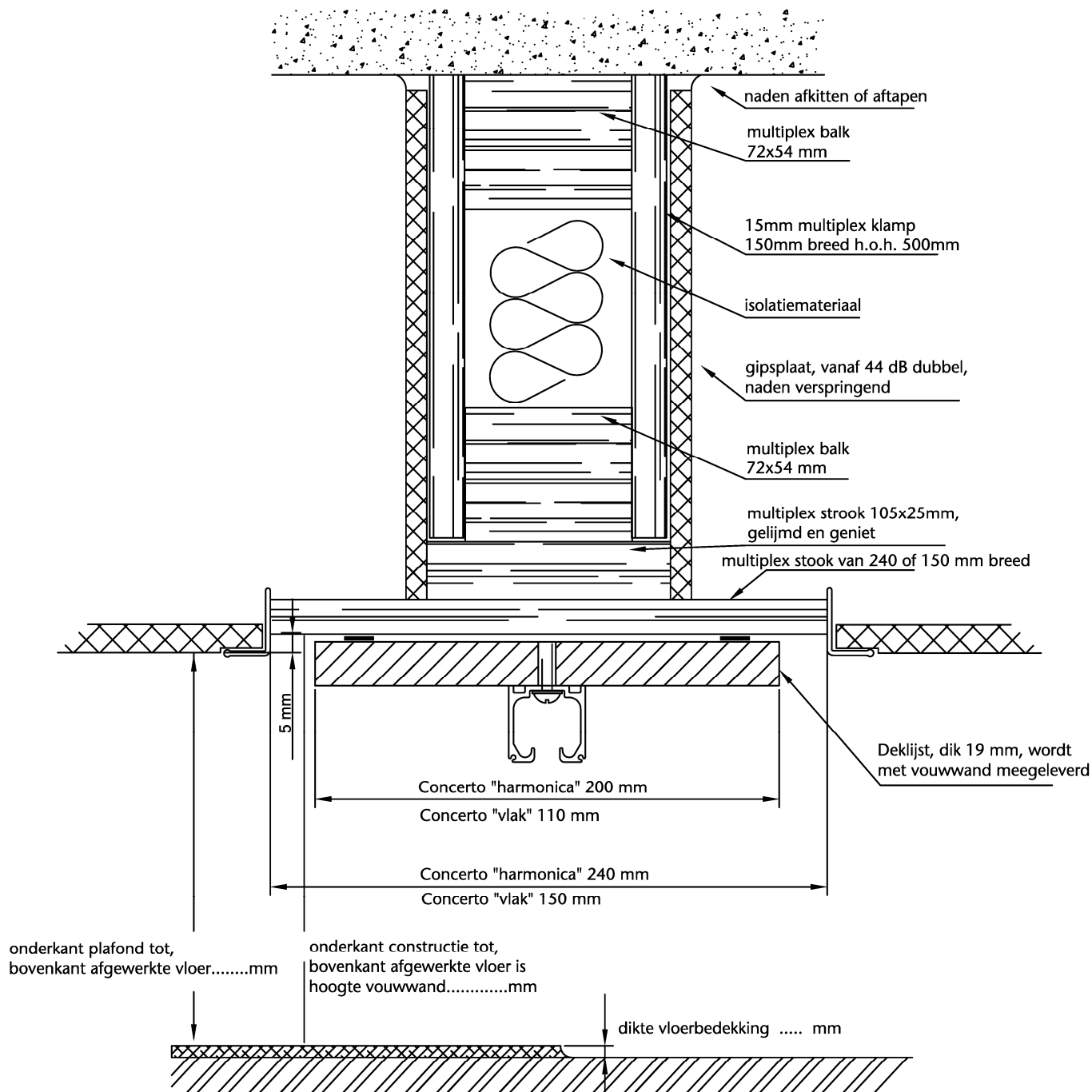
Tekening BVD1
