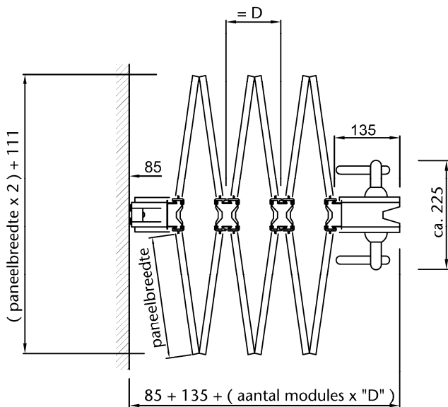
Tekening VD3
