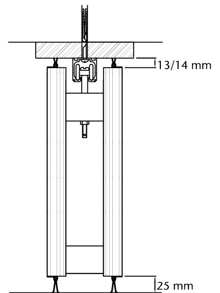
Tekening VD4
