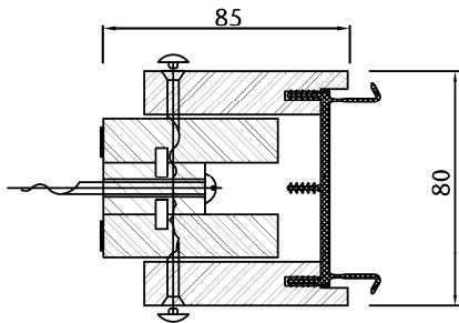
Tekening VD1
