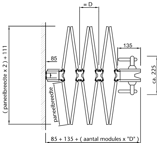
Tekening VD3
