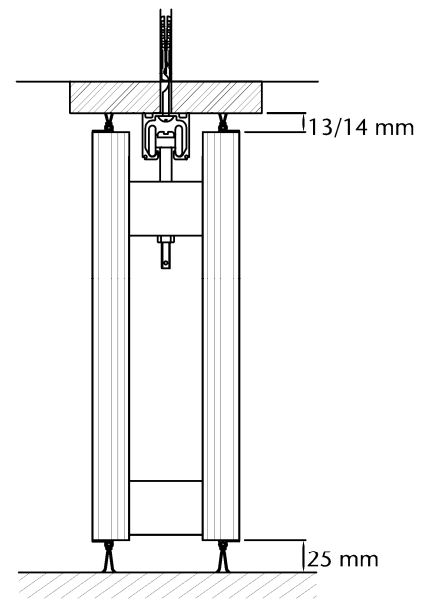
Tekening VD4
